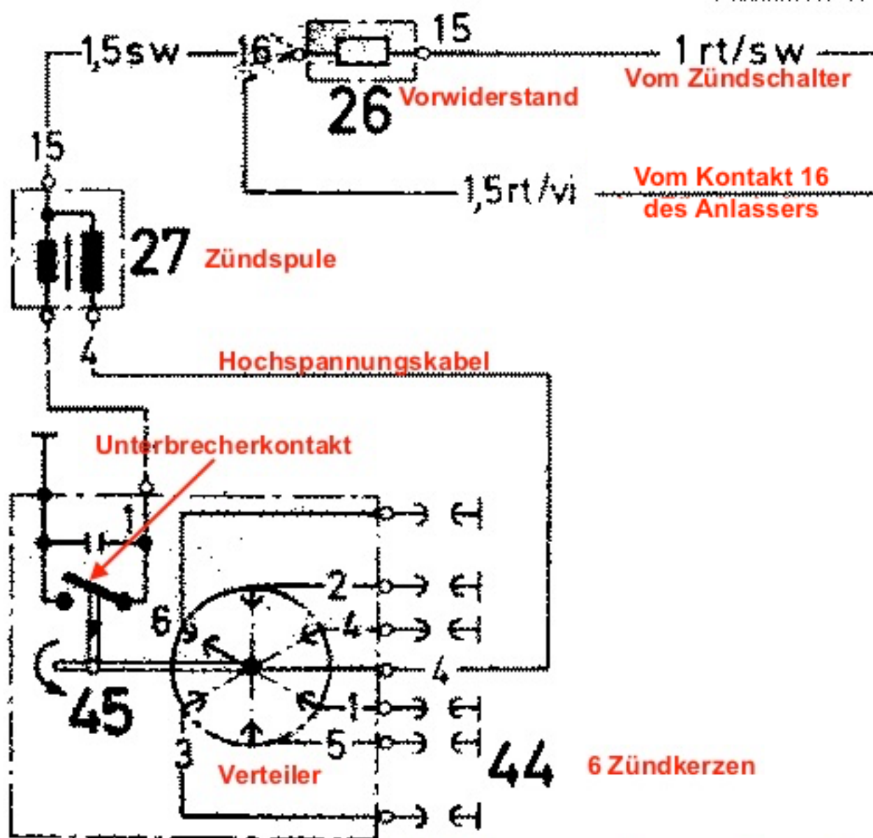
Zündkomponenten an einem 230.6er, 250er, 250C (Dez. 1970 - Mai 1972)
